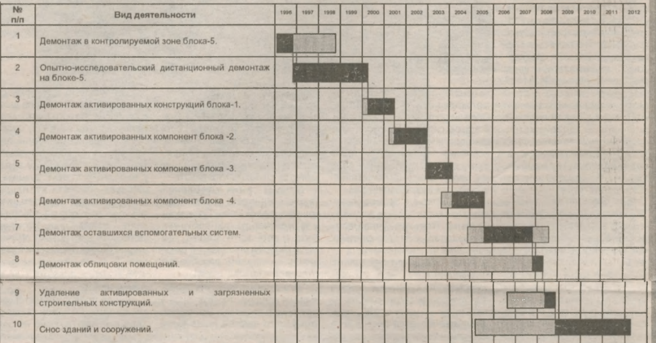
Рис.4. Базовый график выполнения работ по снятию с эксплуатации АЭС "НОРД"
