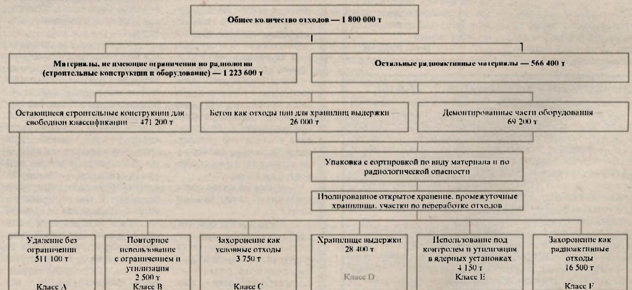
Рис.3. Ожидаемые потоки материалов при снятии АЭС Грайфсвальда с эксплуатации
