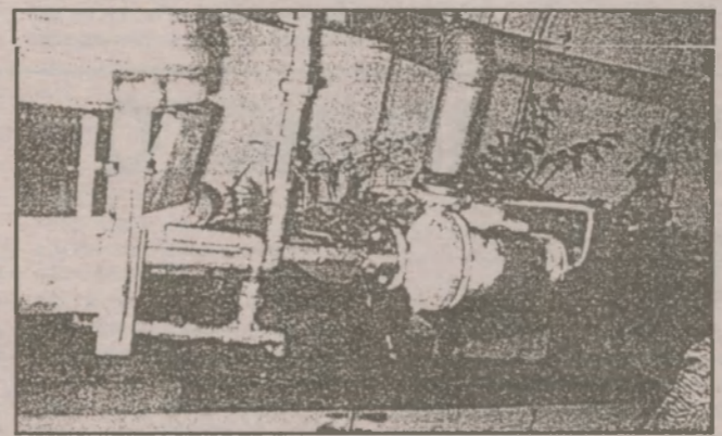
Трубопровод системы охлаждения осадительного блока, из которого была дренирована вода, чтобы подавить критическую ценную ядерную реакцию деления.
